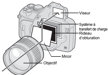
Prise de vue à l'aide du viseur
