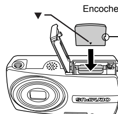
Couvercle de la carte/du compartiment de la batterie
