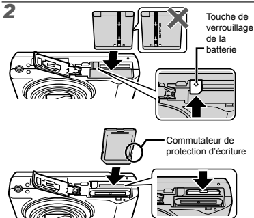
Verrou du compartiment de la batterie/carte
