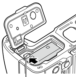
Perilla de bloqueo de la batería
